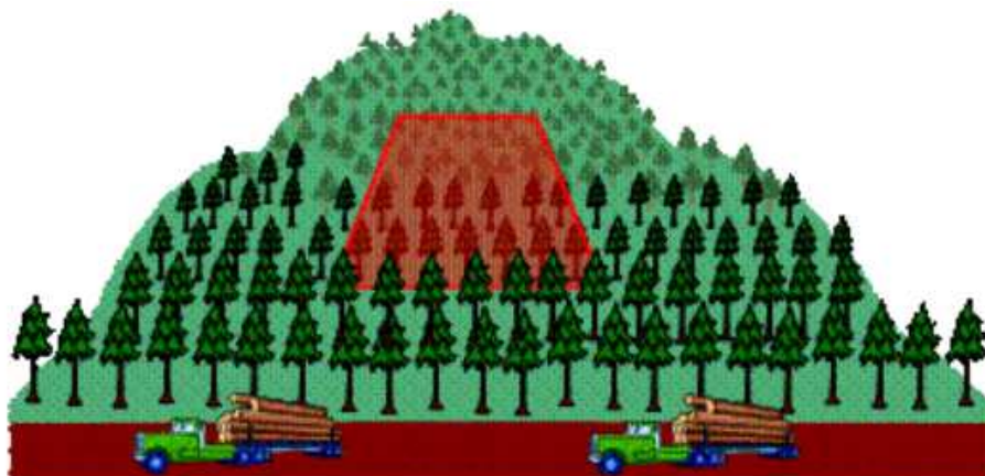
図4 プロジェクト実施地に傾斜がある場合のモニタリングプロット設定方法 ※赤部は設定したプロットを示す。
